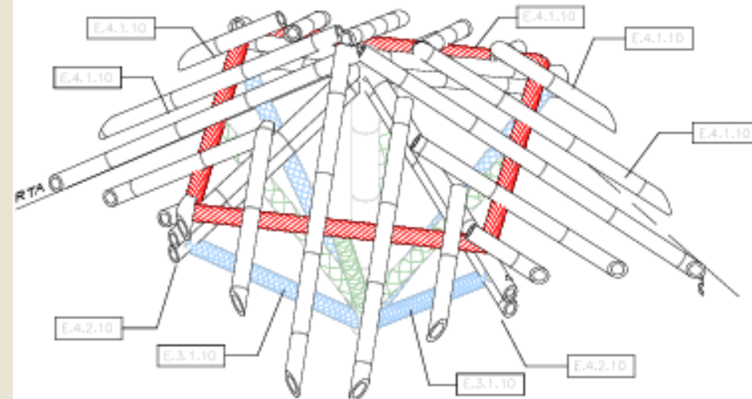
5 AXONOMETRIA Z-1
